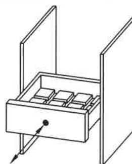
Схема испытания на долговечность
